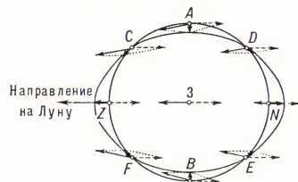
Распределение приливообразующих сил в различных точках (А, В, С, ...) поверхности Земли, вызванных притяжением Луны; тонкие стрелки — силы притяжения, пунктирные — вычитаемая сила притяжения в центре Земли, жирные — приливные силы.
